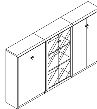
VID212C 2514x380x1400
